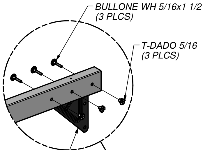
TRIANGOLO PIATTO BLU 100 5 BUCO
