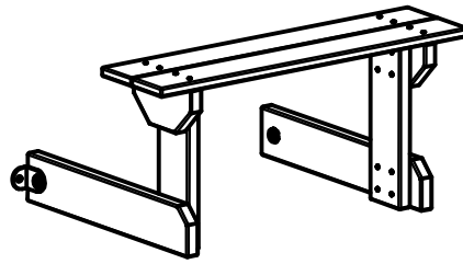
ASSEMBLAGGIO PANCA
