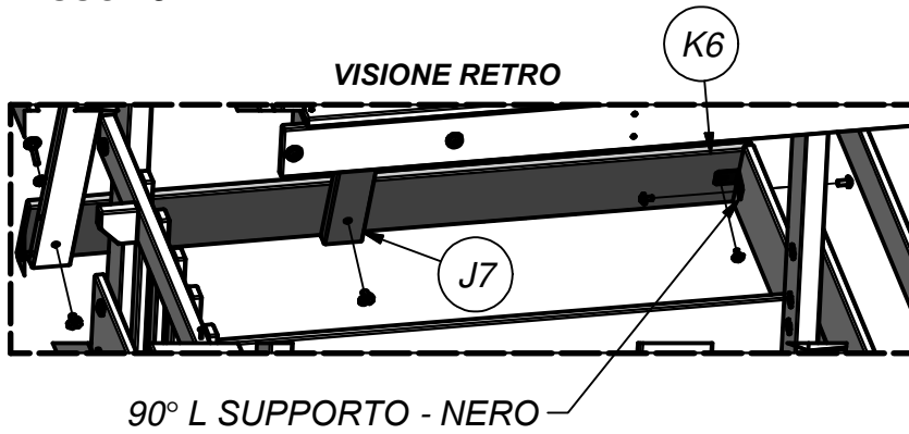
(1) - 90° L SUPPORTO - NERO- A4M00555
