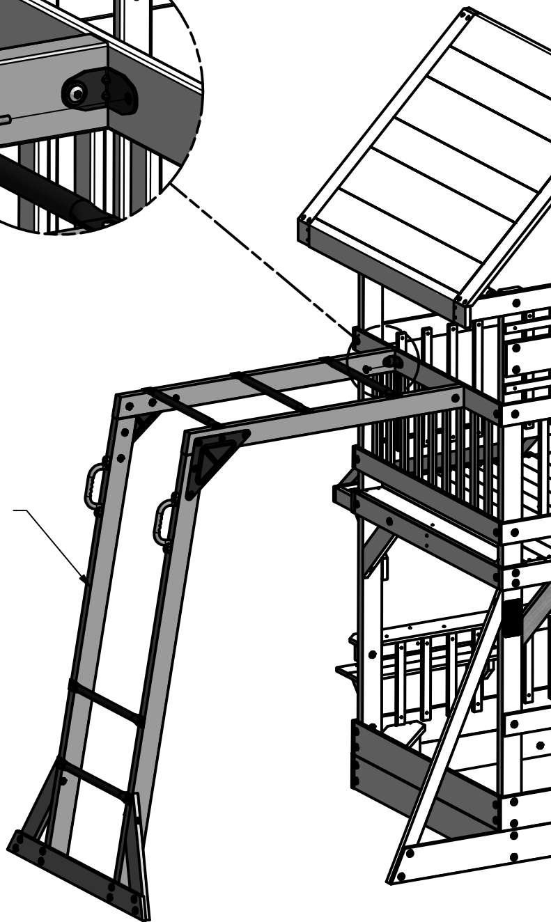
ASSEMBLAGGIO MONKEY BAR
